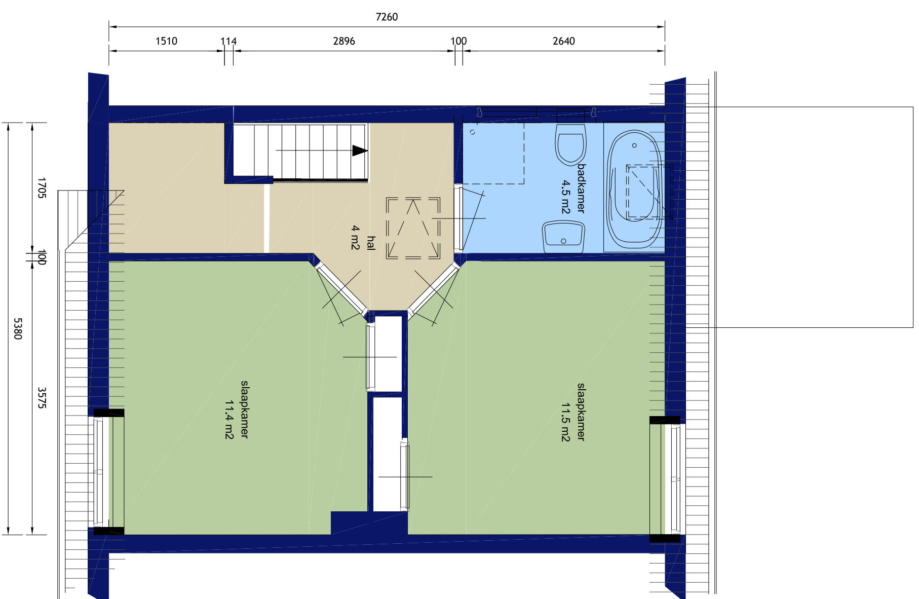
1e verdieping
