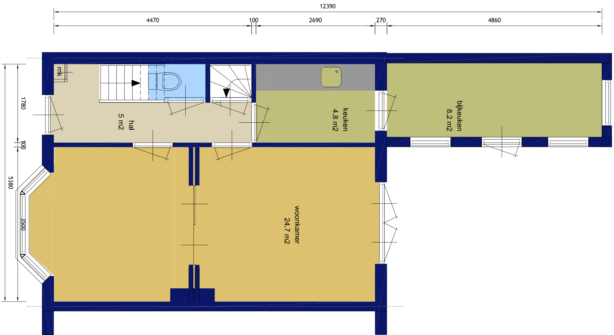
begane grond
