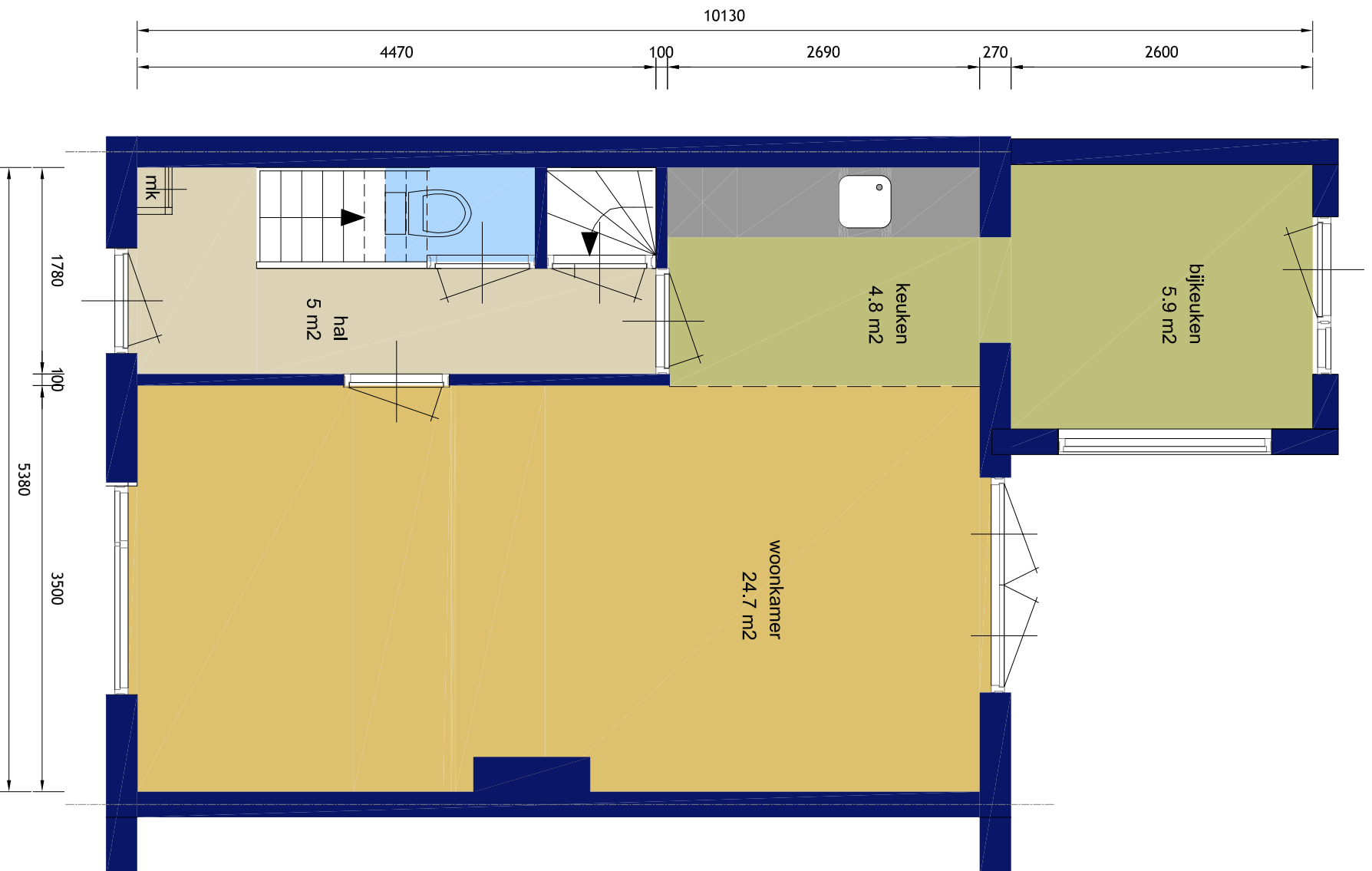
begane grond
