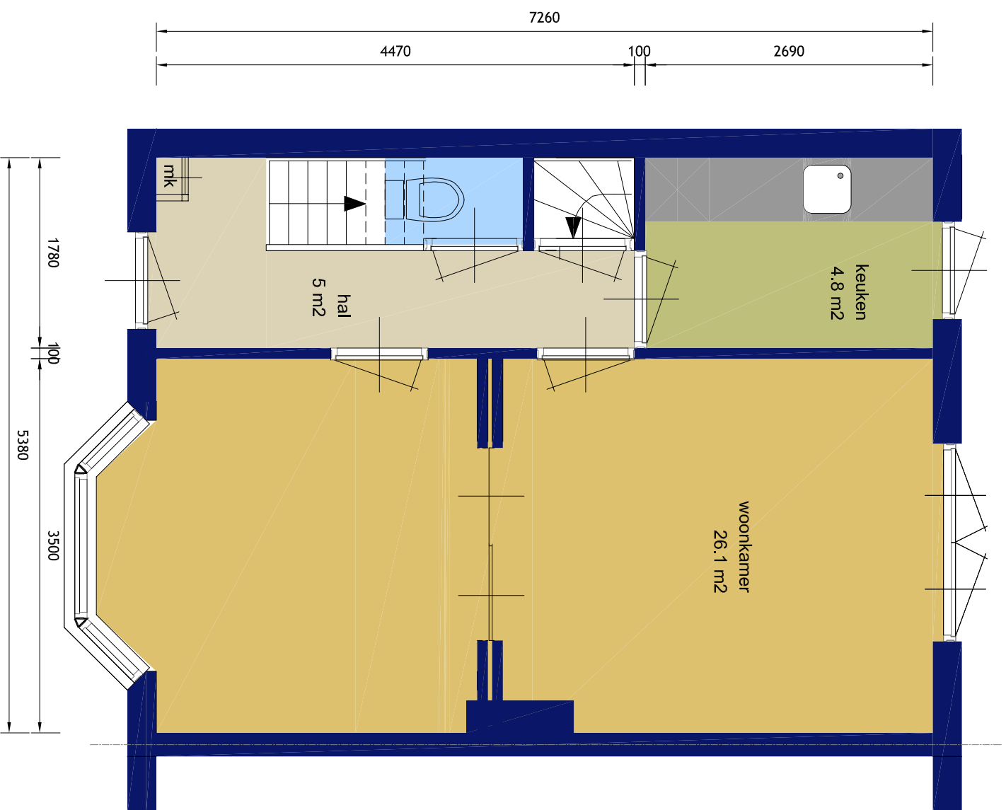
begane grond
