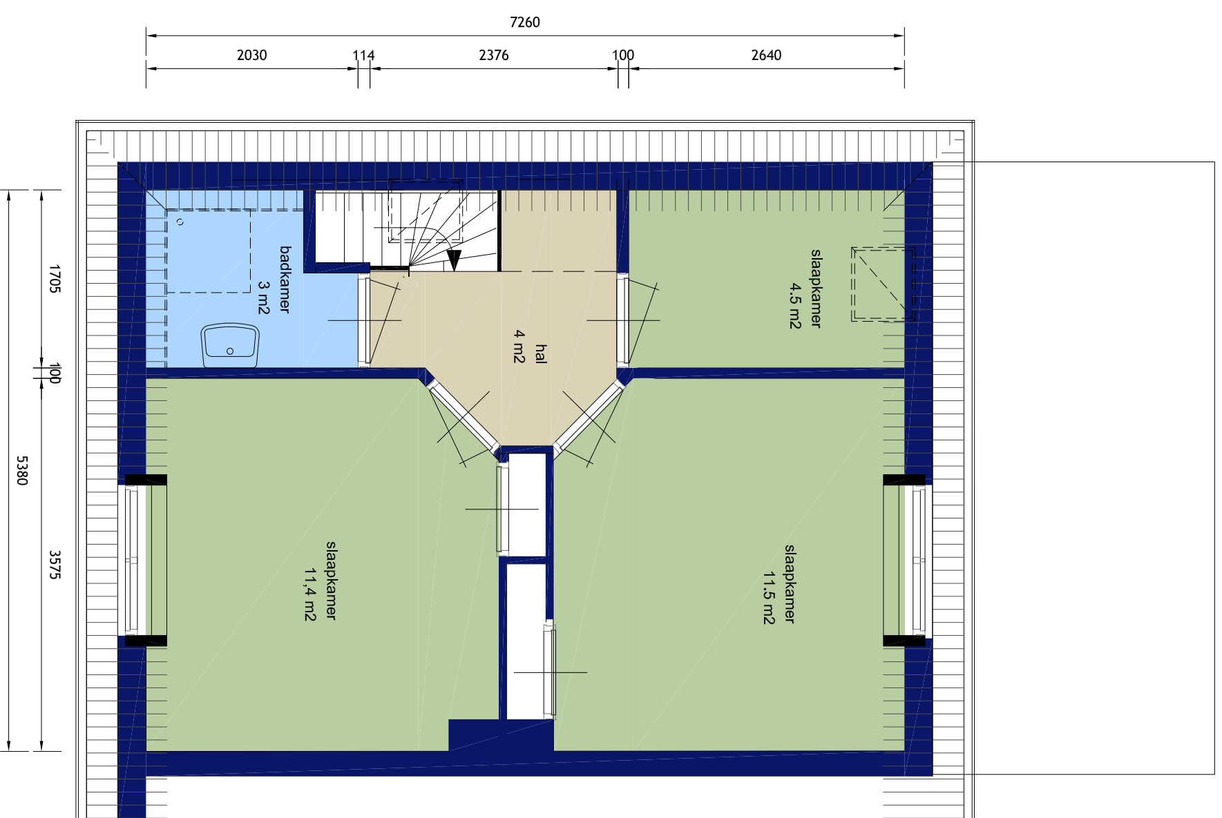
1e verdieping
